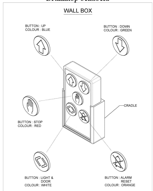
Radiografische drukknop
