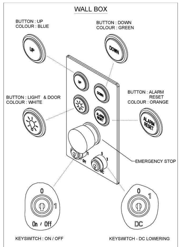
Drukknop bekabeld
